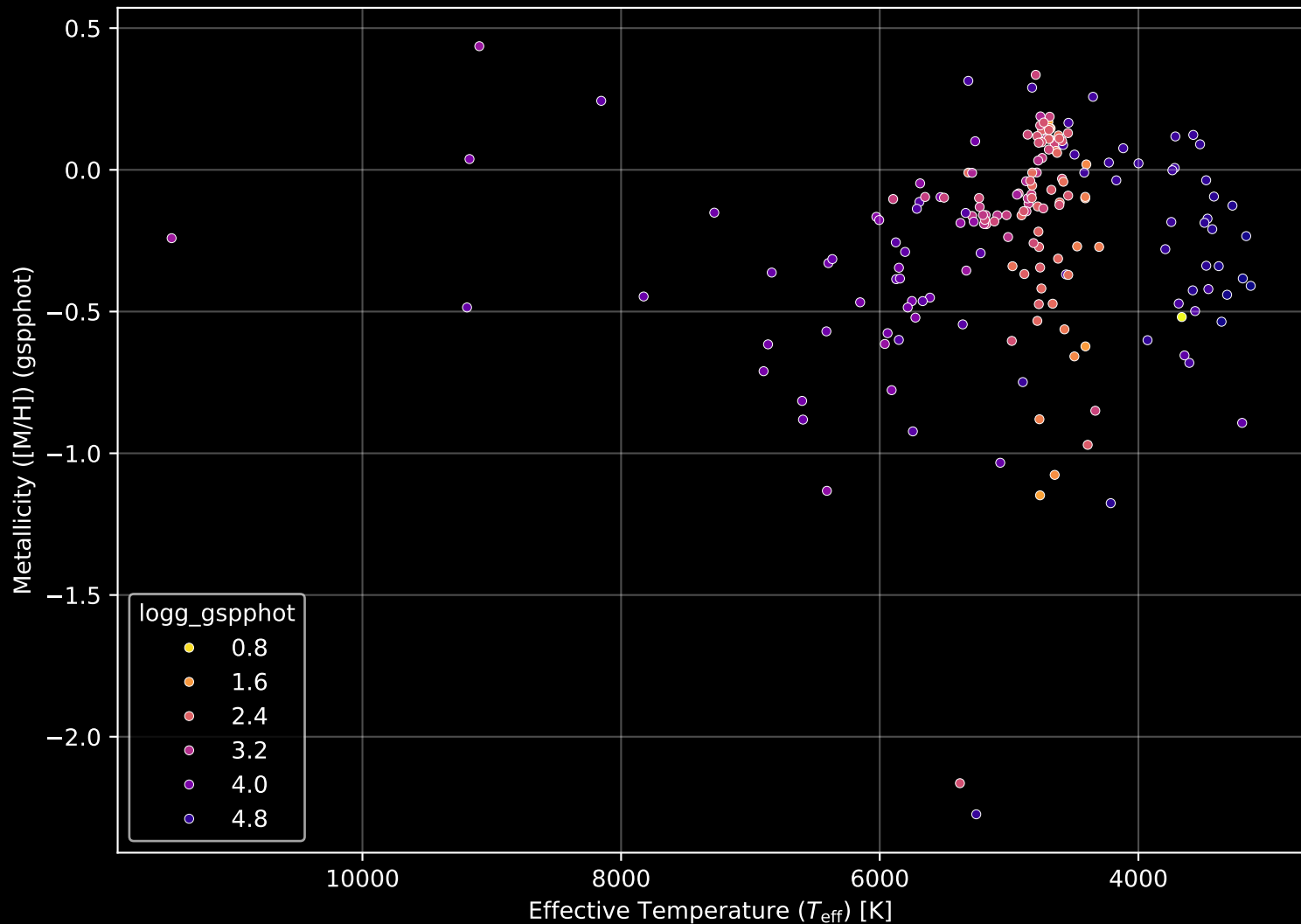
APOGEE DR17 Field: [K2_C7_010-14_btx] Stellar Population Parameters (n= 183)
